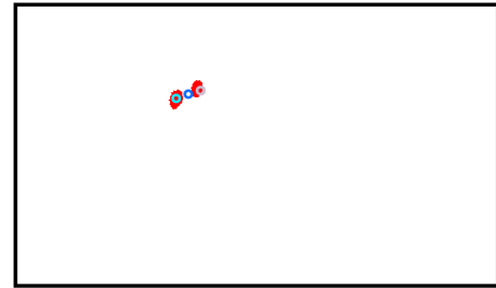
図 4: 塊検出結果
