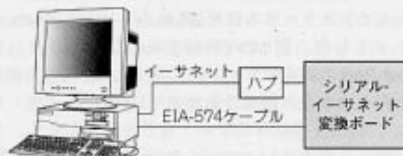
〈図12〉簡単な通信テストを行うための接続
