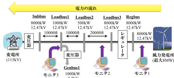
図 2: 基本的な風力発電の配電網
