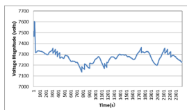
図 4: モニタ 1 電圧
