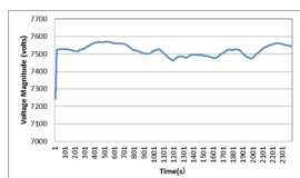
図 5: モニタ 2 電圧
