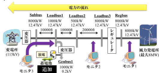
図 7: 蓄電池を追加した風力発電の配電網
