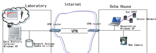
図 1: センサネットワーク実験環境
