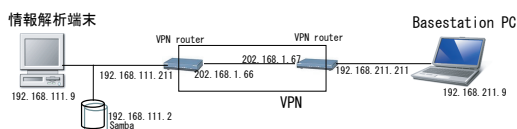
図 4: VPN を経由しリモートからデータを観測
