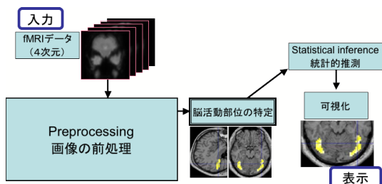
図 1: 解析の流れ
